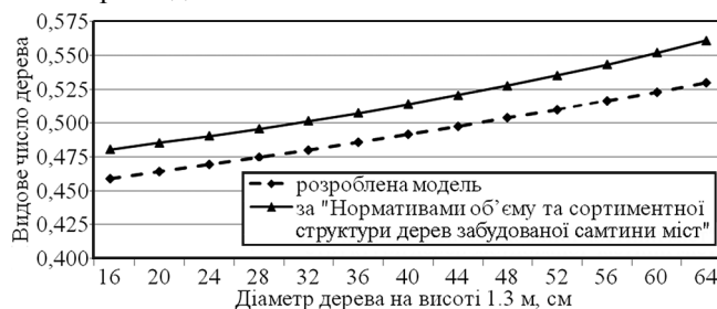
Рис. 1. Графічна ілюстрація моделей видового числа
